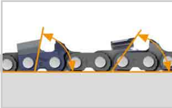
Различные передние углы
